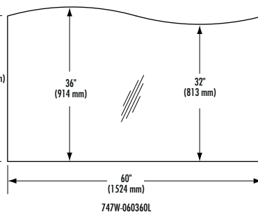
747W-060360L
